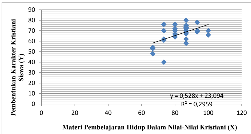
Gambar 1. Kurva Persamaan Regresi Sederhana X (Penguasaan Materi Pembelajaran Hidup Dalam Nilai-Nilai Kristiani ) Terhadap Y (Pembentukan Karakter Kristiani Siswa)
